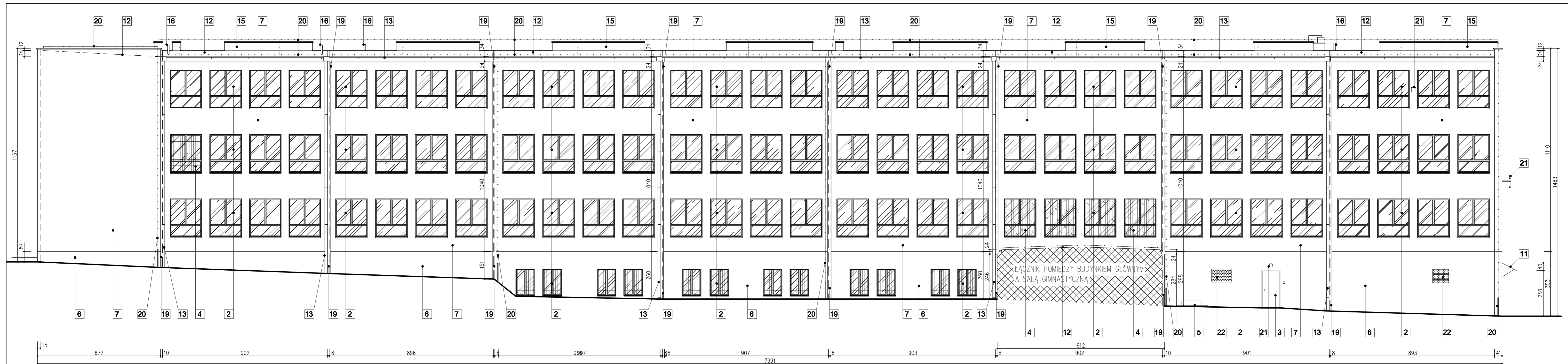
ELEWACJA POŁUDNIOWA (BUDYNEK GŁÓWNY)
